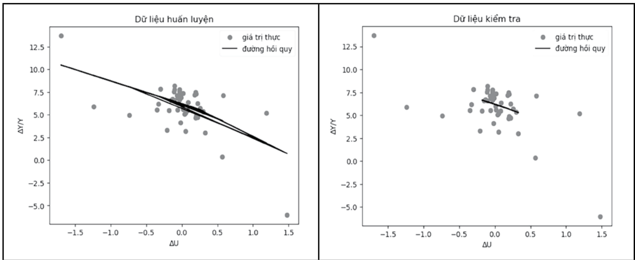
Hình 3. Mô hình hồi quy Keras với bộ dữ liệu huấn luyện và kiểm tra
